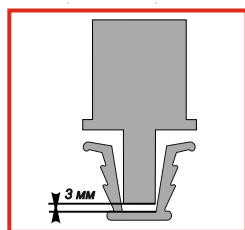
Регулировка створок.
