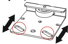
Регулировка створок.
