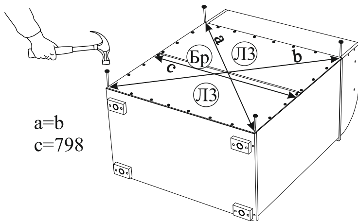
Рис.9 Схема прибивки ЛДВП
