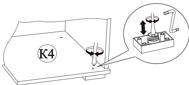
Рис.8 Регулировка опор
