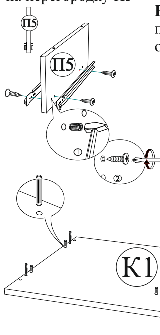
Рис.1 Прикручивание направляющих
