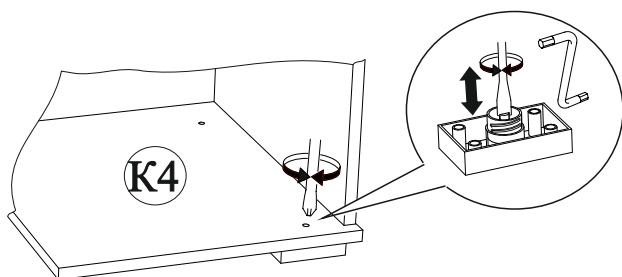
Рис.7 Регулировка опор
