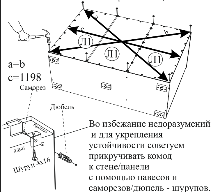
Рис.7 Прибивка ЛДВП
