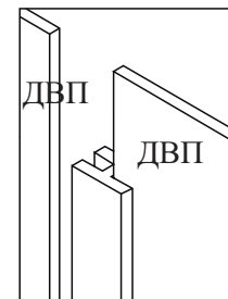
Установка соединителя ДВП
