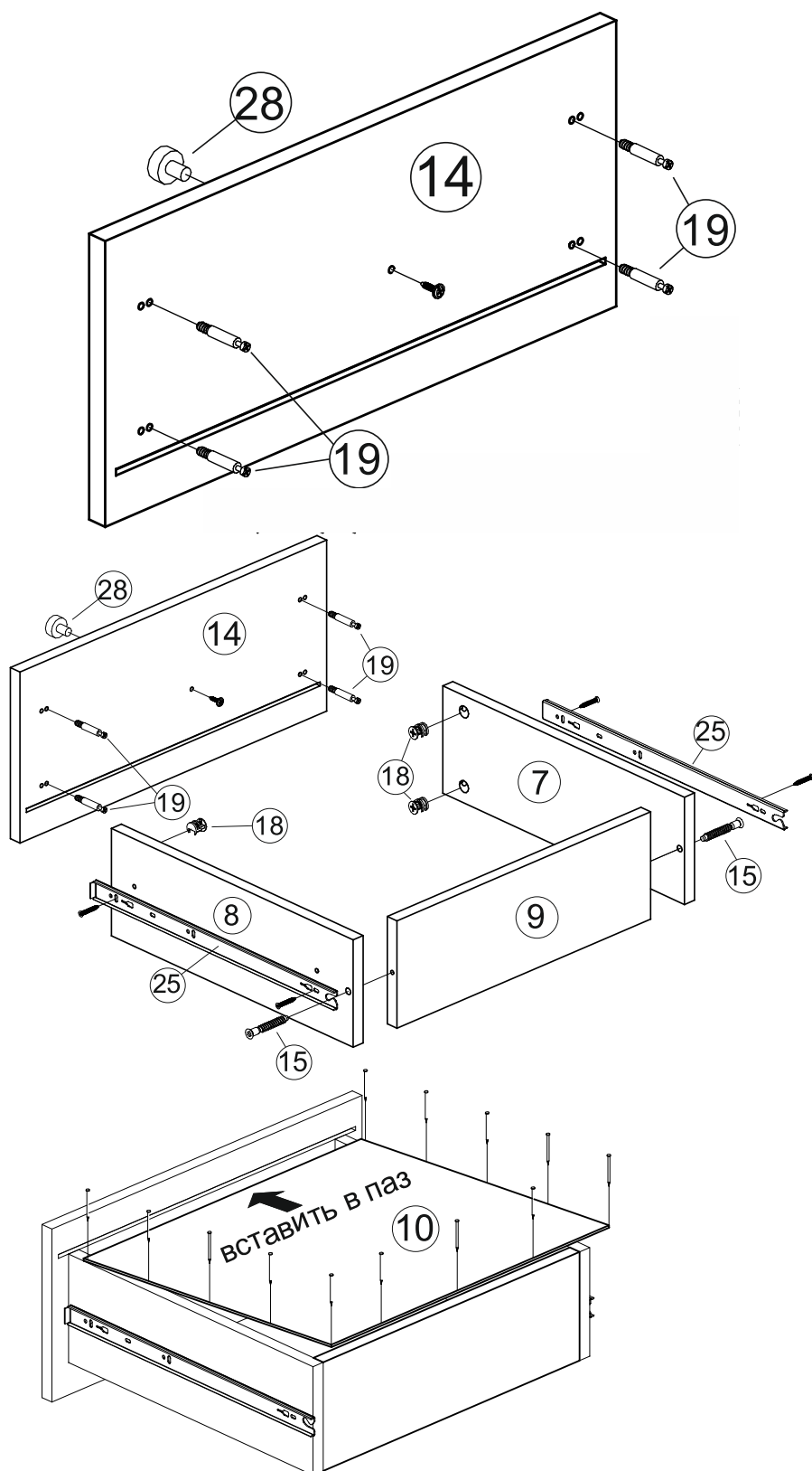
Рис.8 Сборка ящика
