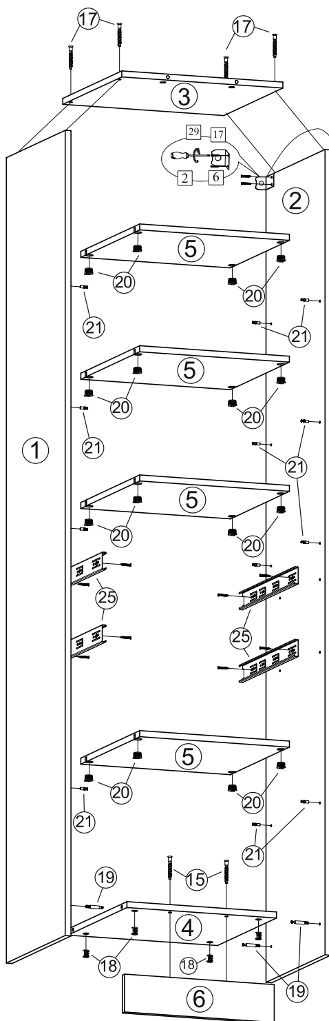
Рис.1 Сборка каркаса
