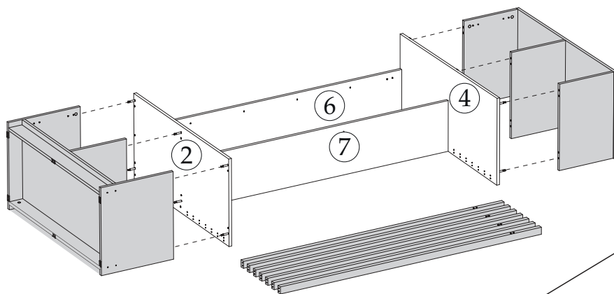
Левосторонняя сборка
