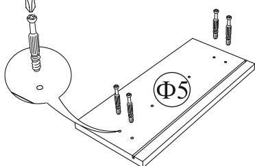
Рис.8 Порядок сборки выдвижного ящика
