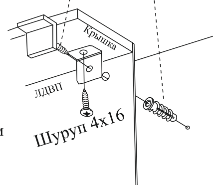
Дюбель
