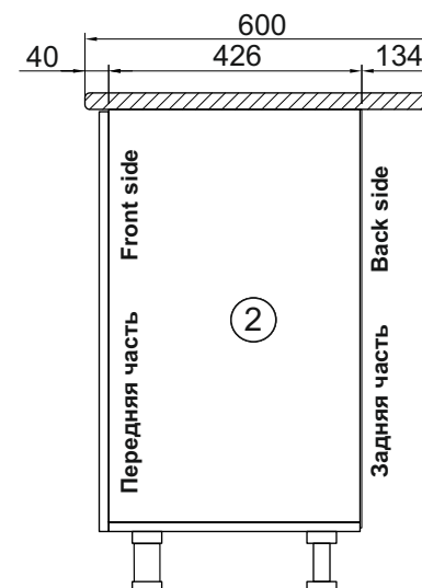
Установка столешницы (вид сбоку)
