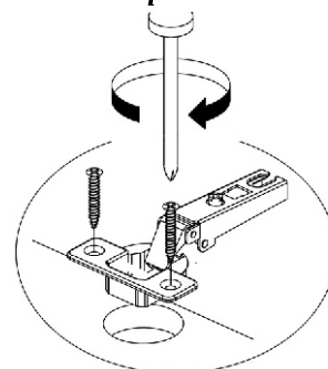
Рис.10 - Монтаж чашки втли 36б на фасад
