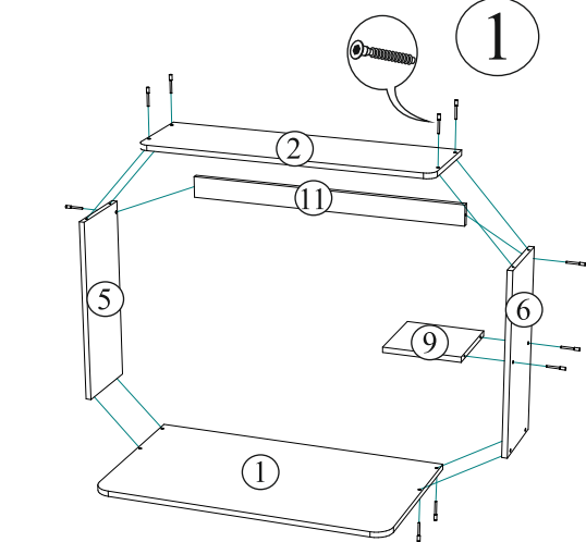
Рис.1 - Схема сборки надстройки компьютерного стола
